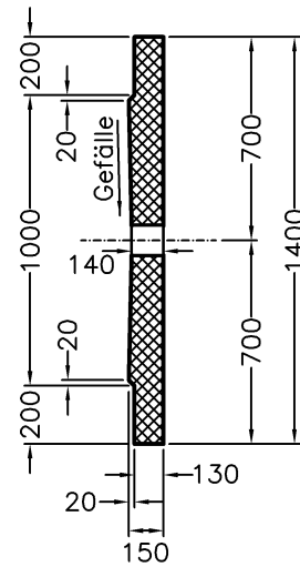
Querschnitt
