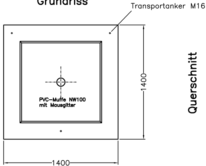
Grundriss
