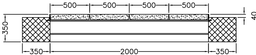
Querschnitt
