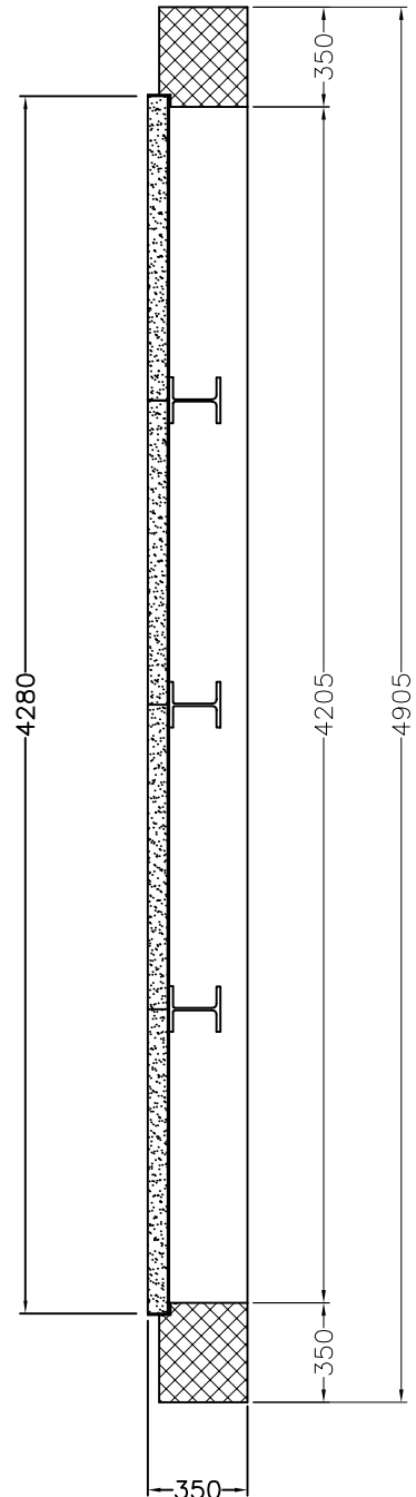
Längsschnitt
