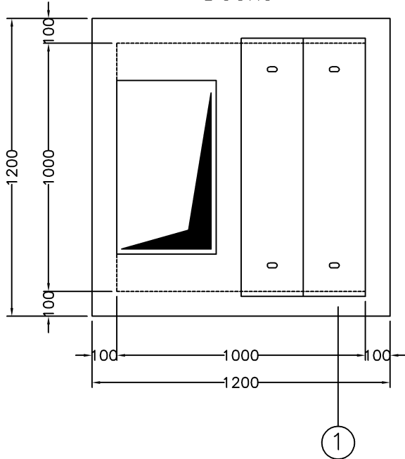
Grundriss Decke
