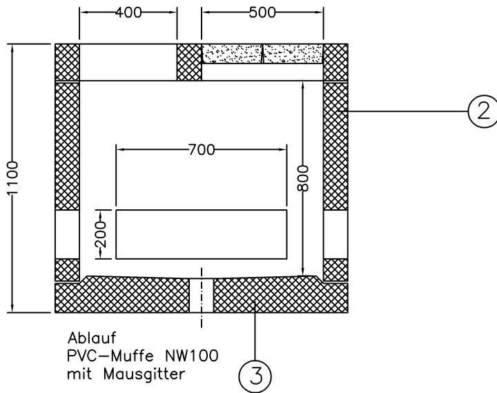
Querschnitt
