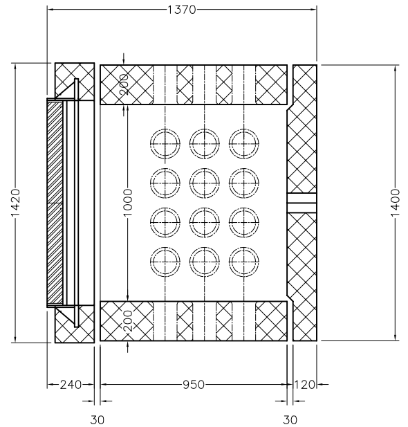
Längsschnitt
