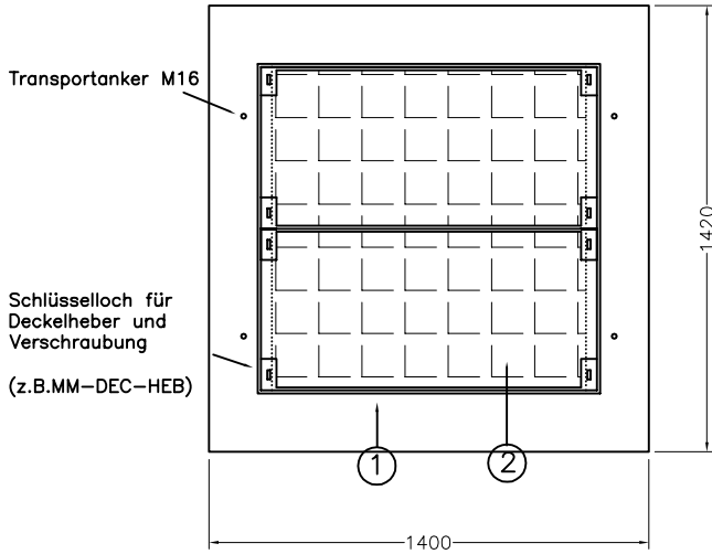
Grundriss
