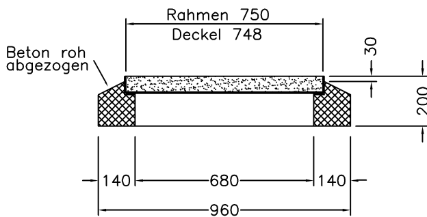
Querschnitt
