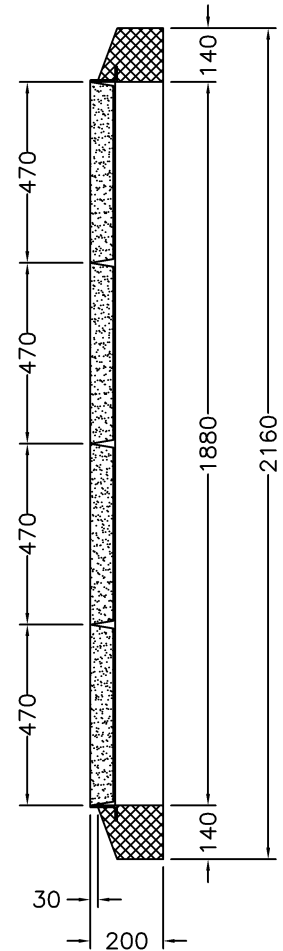
Längsschnitt
