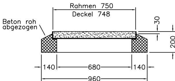
Querschnitt
