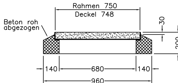
① ② Querschnitt
