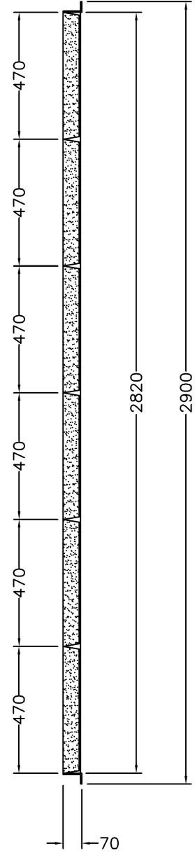
Längsschnitt
