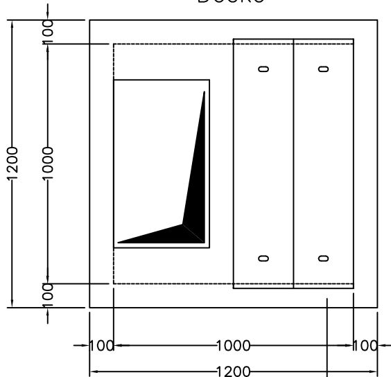
Grundriss Decke
