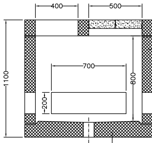
Querschnitt
