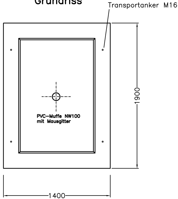
Grundriss
