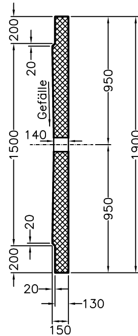
Querschnitt
