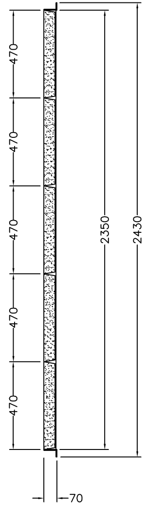
Längsschnitt
