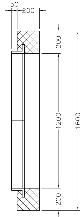
Längsschnitt
