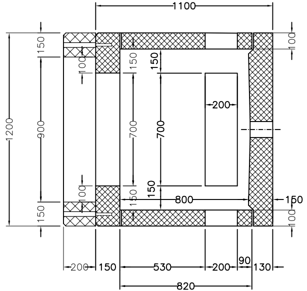
Längsschnitt
