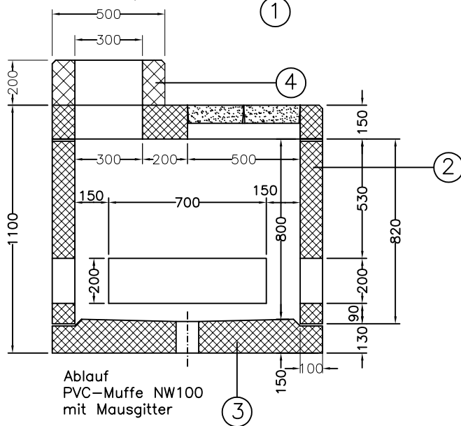
Querschnitt
