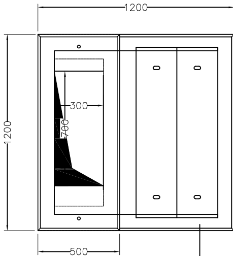
Grundriss Decke
