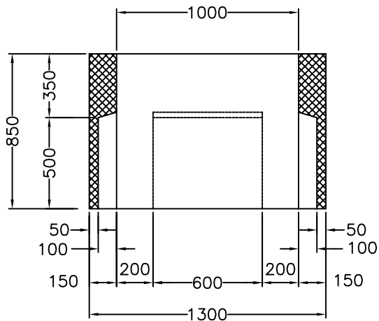
Querschnitt
