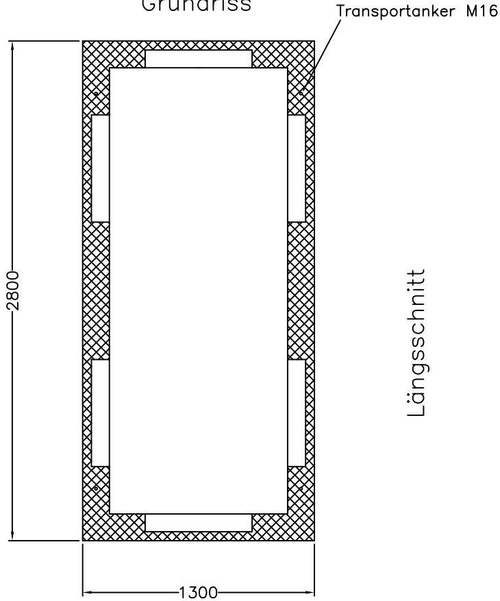
Grundriss
