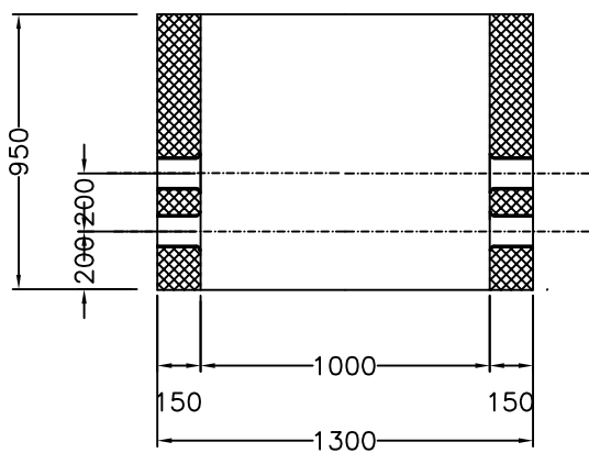
Längsschnitt
