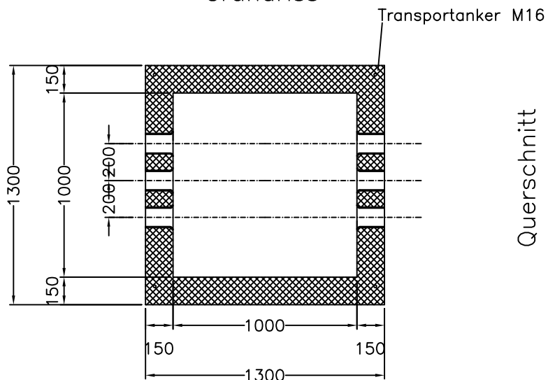
Grundriss
