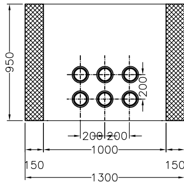
Querschnitt
