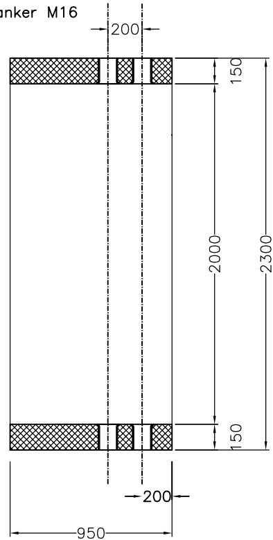
Längsschnitt
