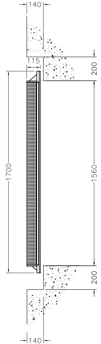
Längsschnitt
