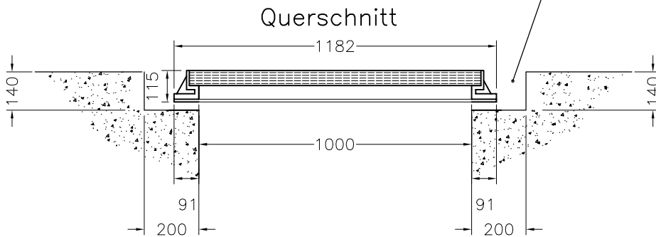
empfohlene Aussparung
