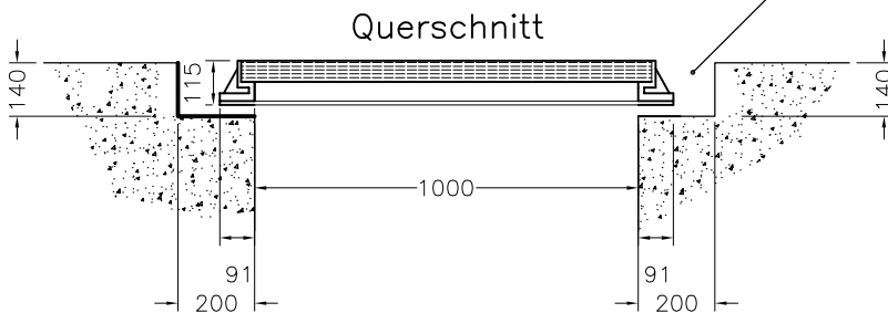
empfohlene Aussparung
