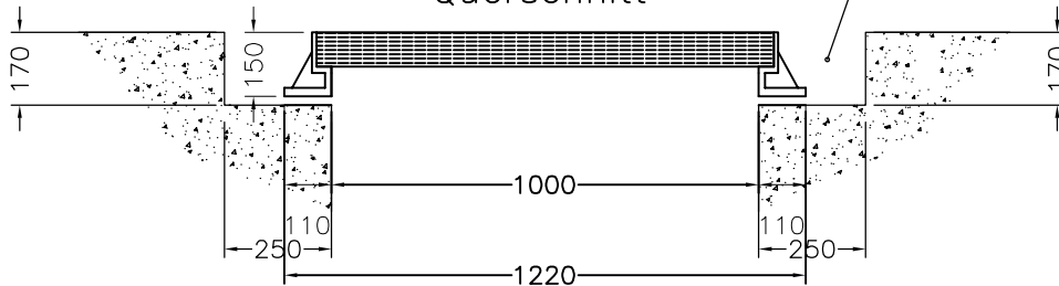
Querschnitt
