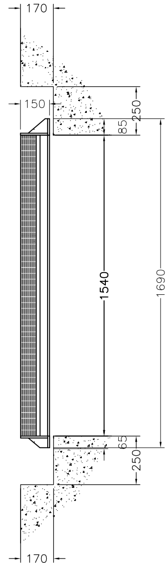
Längsschnitt
