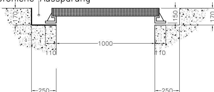
empfohlene Aussparung
