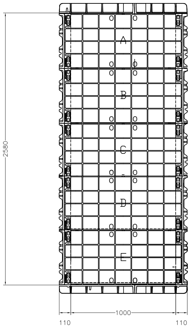
empfohlene Aussparung
