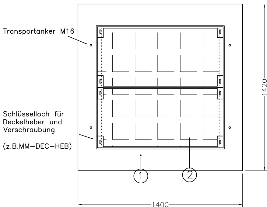
Grundriss
