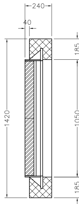
Längsschnitt
