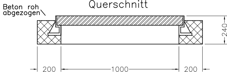
Querschnitt
