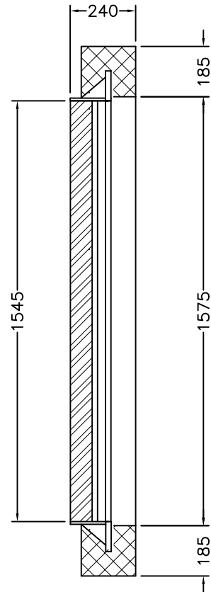
Längsschnitt
