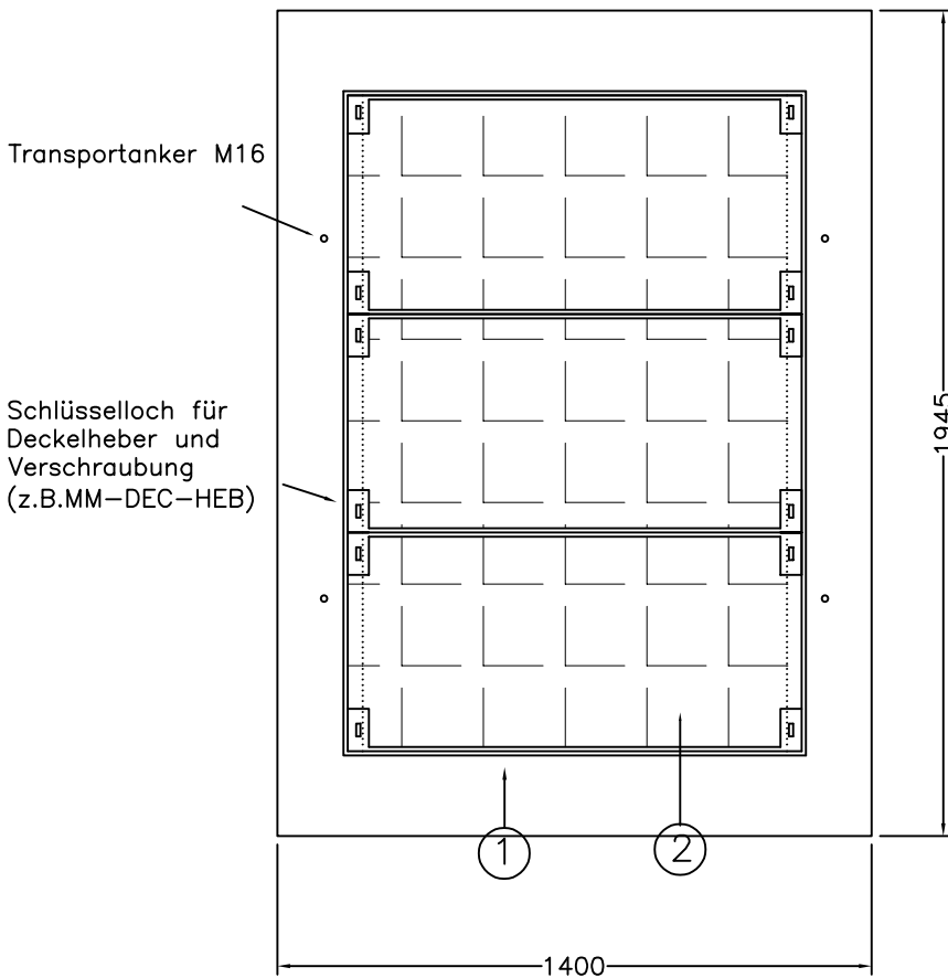
Grundriss
