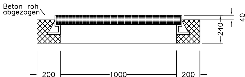
Querschnitt
