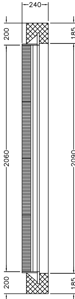
Längsschnitt
