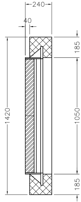
Längsschnitt
