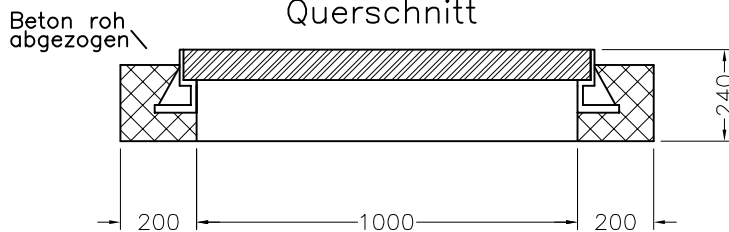
Querschnitt
