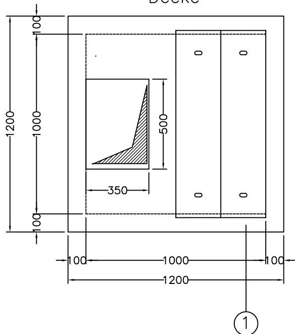
Grundriss Decke
