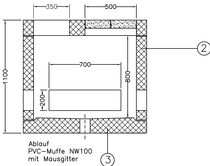
Querschnitt
