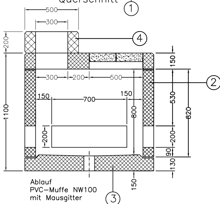
Querschnitt
