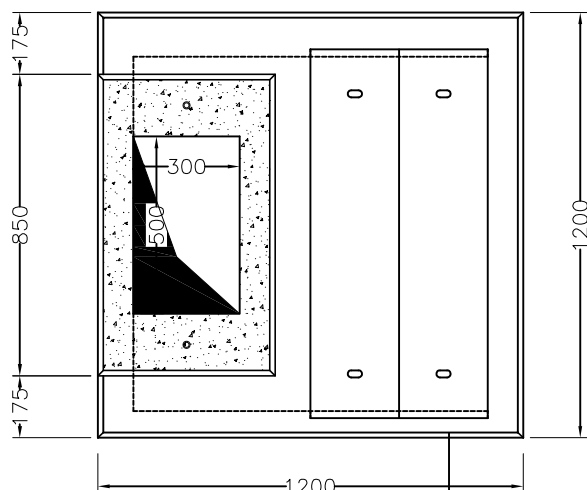
Grundriss Decke
