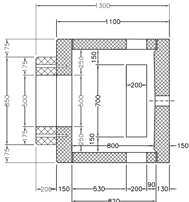
Längsschnitt
