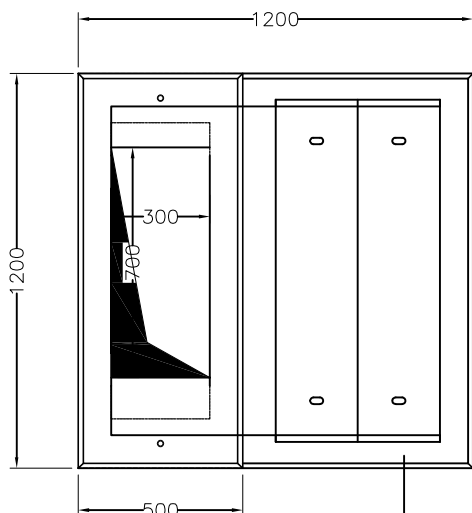
Grundriss Decke
