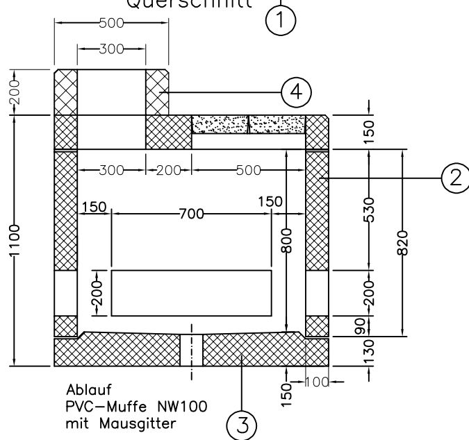
Querschnitt
