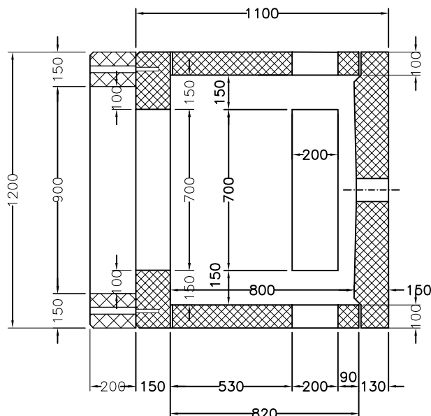
Längsschnitt
